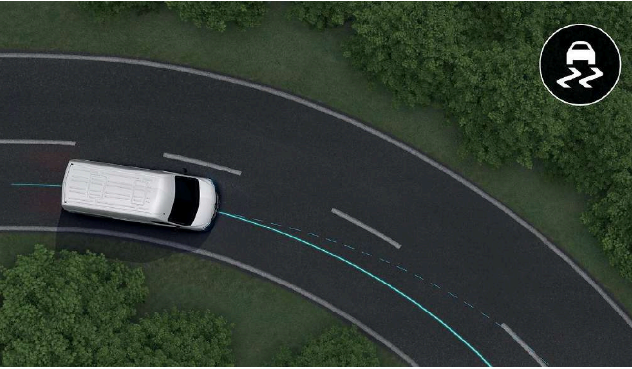
sistema de control de estabilidad (ESP) El ESP permite corregir la trayectoria del vehículo para evitar deslizamientos.
